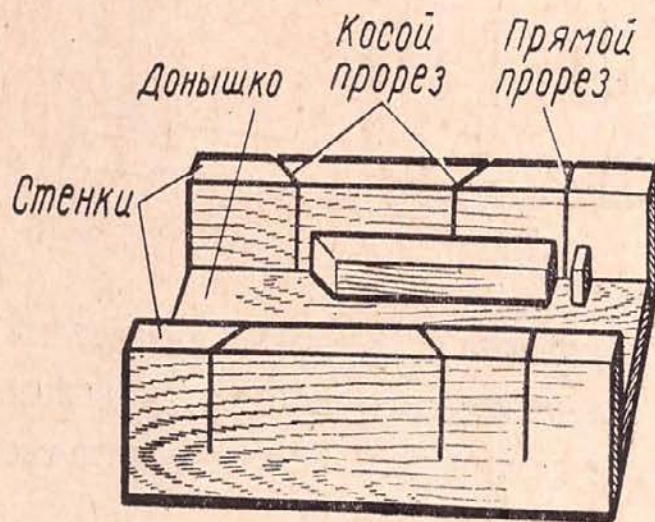
Рисунок 37. Стусло.
