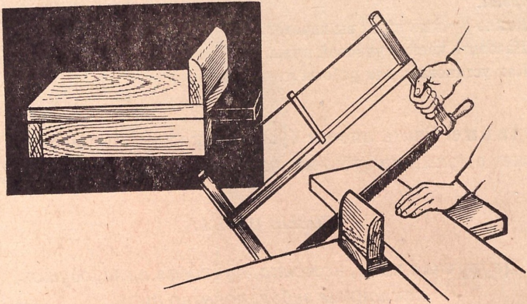
Рисунок 38. Подкладная доска.
